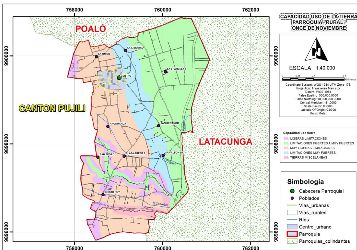
Mapa 20. Capacidad de uso de la tierra.
