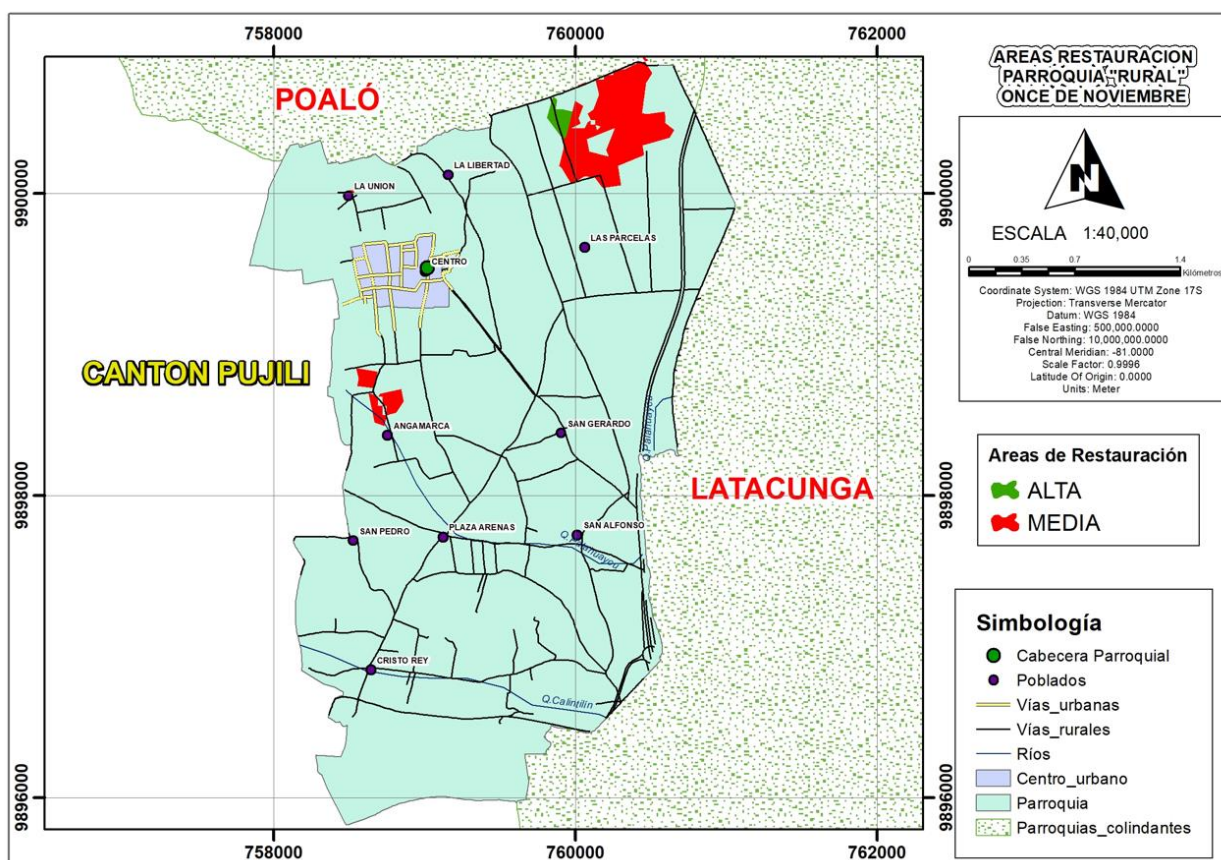
Mapa 15. Áreas para restauración.
