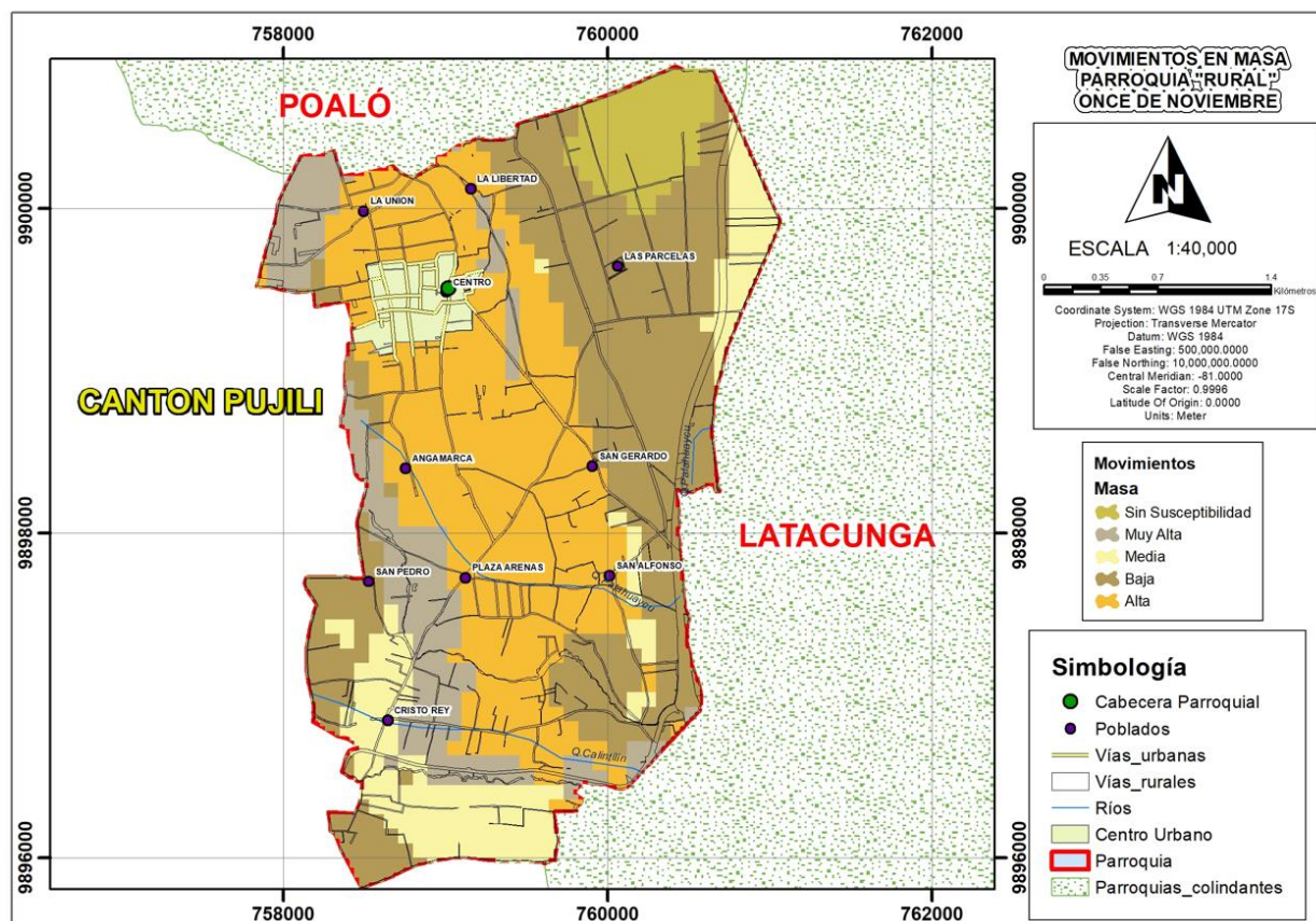
Mapa 6. Movimientos en masa.
